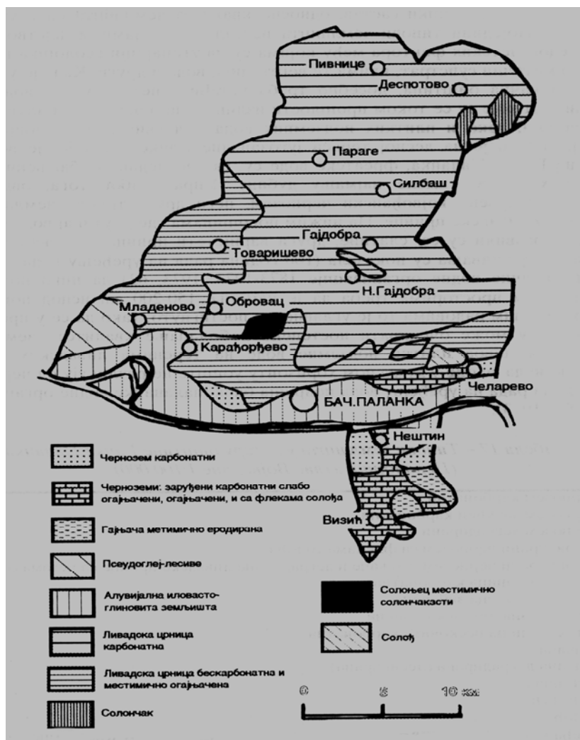
Педеолошка карта бачкопаланачке општине*
